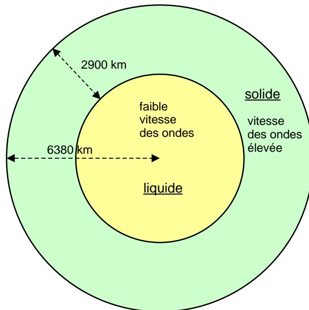
1926 - Modèle de Jeffreys
