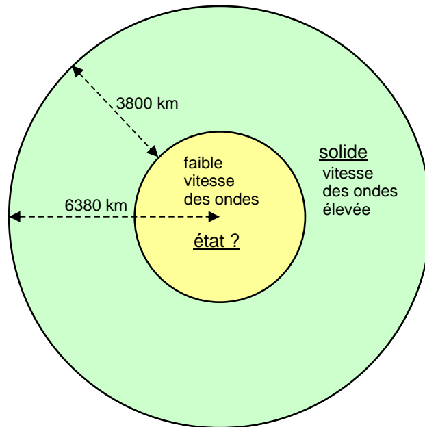
1906 - Modèle de Oldham
