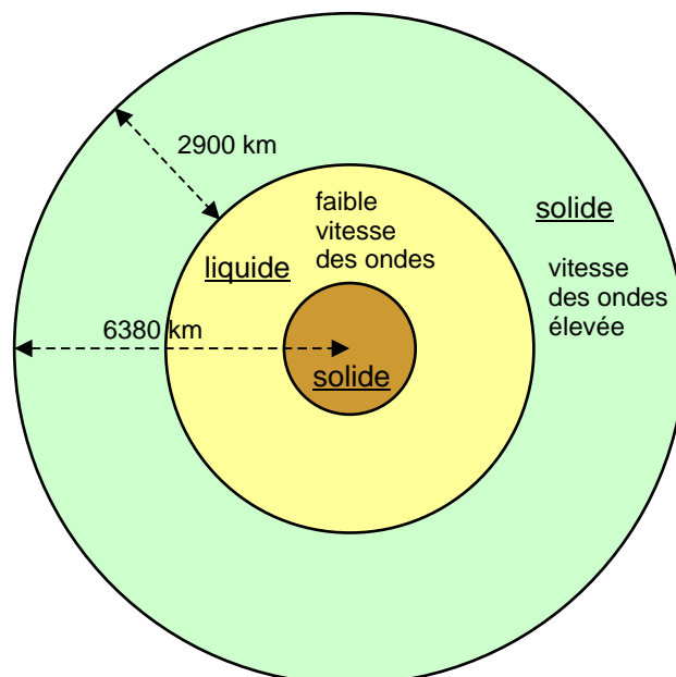
1936 - Modèle de Lehmann
